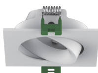
PL-MD18S 83x83x23mm Ø 70mm
