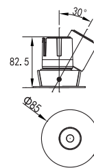
PL-MD45R-9W
